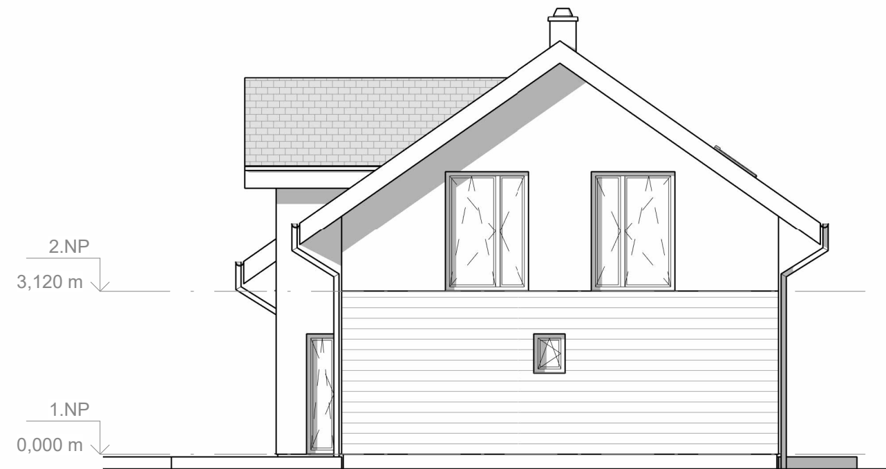
POHĽAD BOČNÝ
