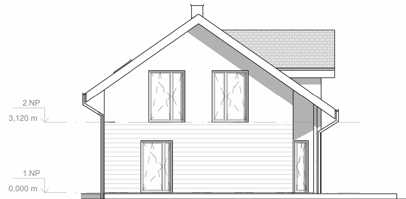
POHĽAD BOČNÝ
